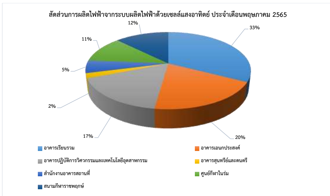
รูปที่ 6 สัดส่วนการผลิตไฟฟ้าของระบบผลิตไฟฟ้าด้วยเซลล์แสงอาทิตย์ ประจำเดือนพฤษภาคม 2565
